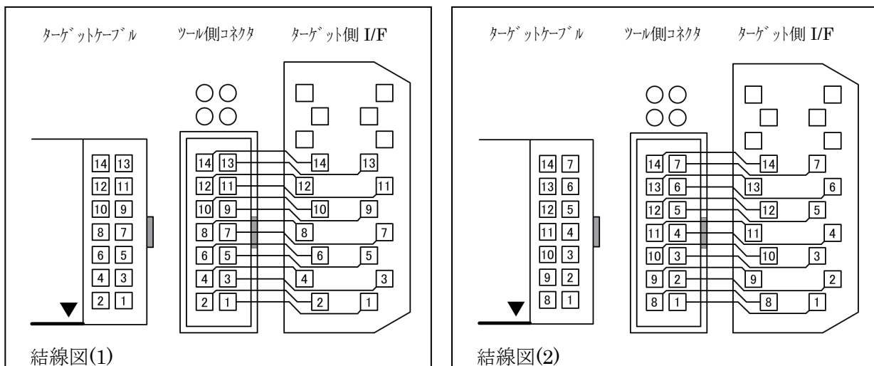
【図5：結線情報】
